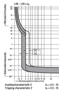
Curva característica Característica Z
