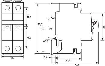
Dibujos acotados Vista de grupos
