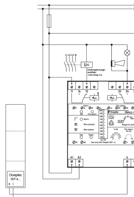
Anschlusschema
