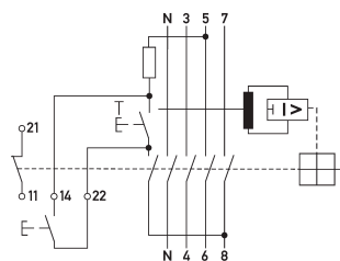
Anschlusschema
